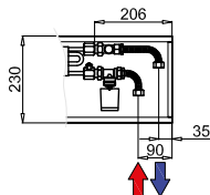
F1S-25 B: 110 mm
